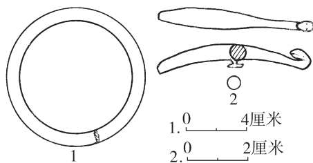
图八 出土铜器
