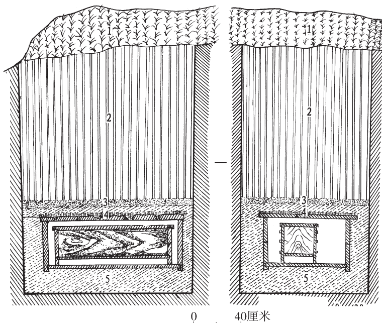
图三 M50 纵、横剖面图
