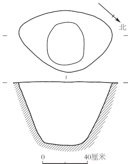
图一— H4 平、剖面图
