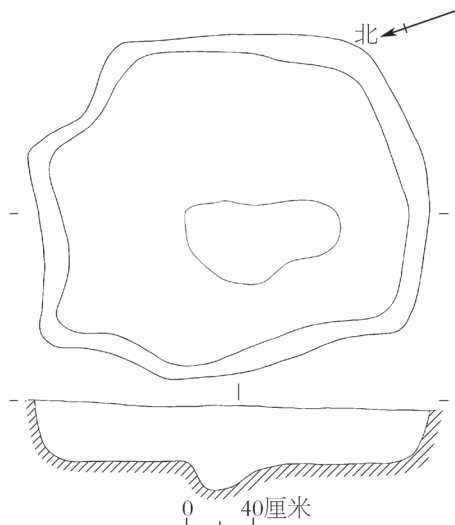
图一四 H27 平、剖面图
