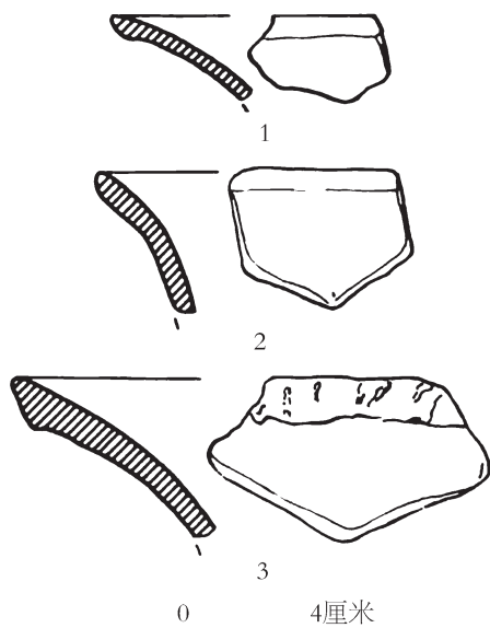
图二〇 III区地层出土泥质陶喇叭口盆
