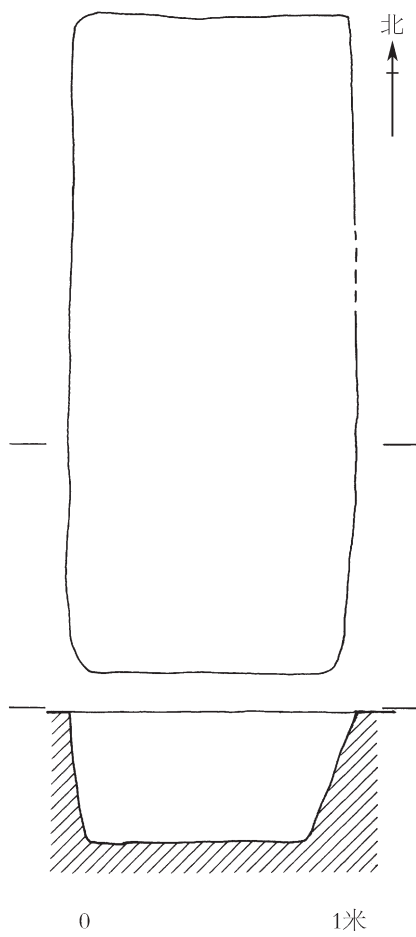
图二二 2010H50 平、剖视图
