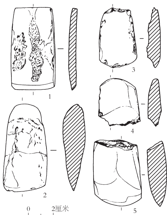
图九 I区地层出土磨制石器
