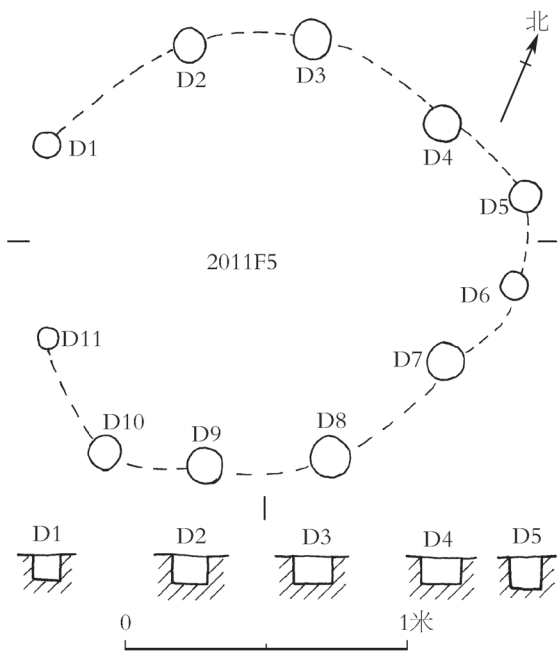
图一五 2011F5 平、剖视图
