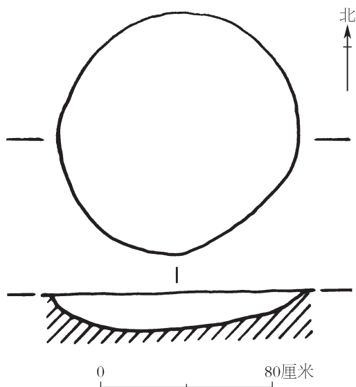
图二三 2012H13 平、剖视图
