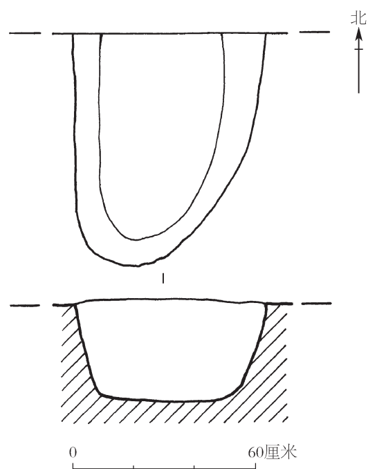
图一〇 2011H33 平、剖视图
