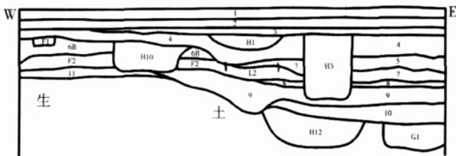
图二十一 T2350 北壁剖面图
