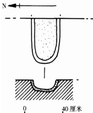
图六 灶(Z1)平、剖面图
