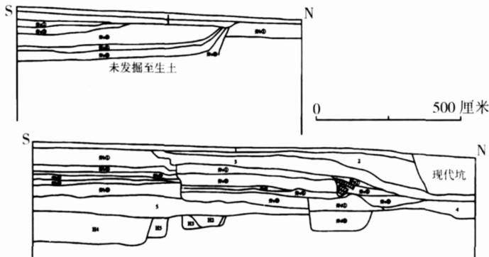
图五 2004MZC I T0805~0809 西壁剖面图
