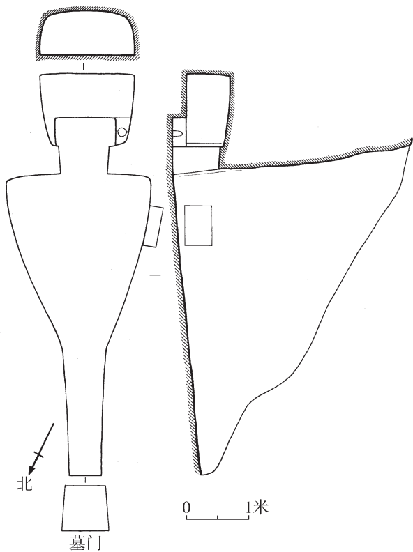
图三 M6 平、剖面图
