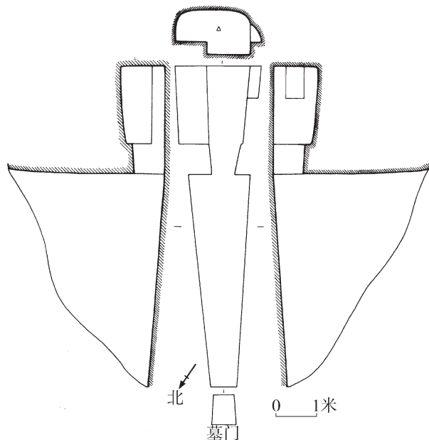
图六 M2平、剖面图
