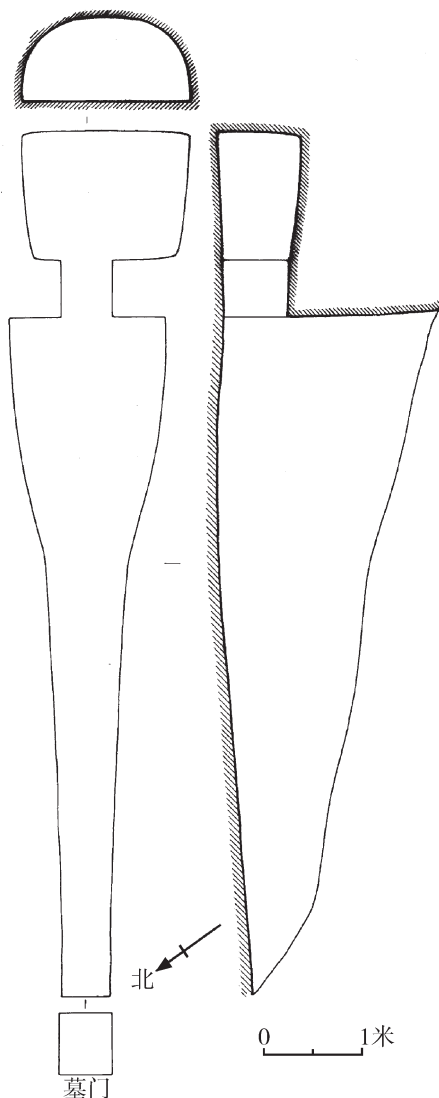
图一〇 M5平、剖面图
