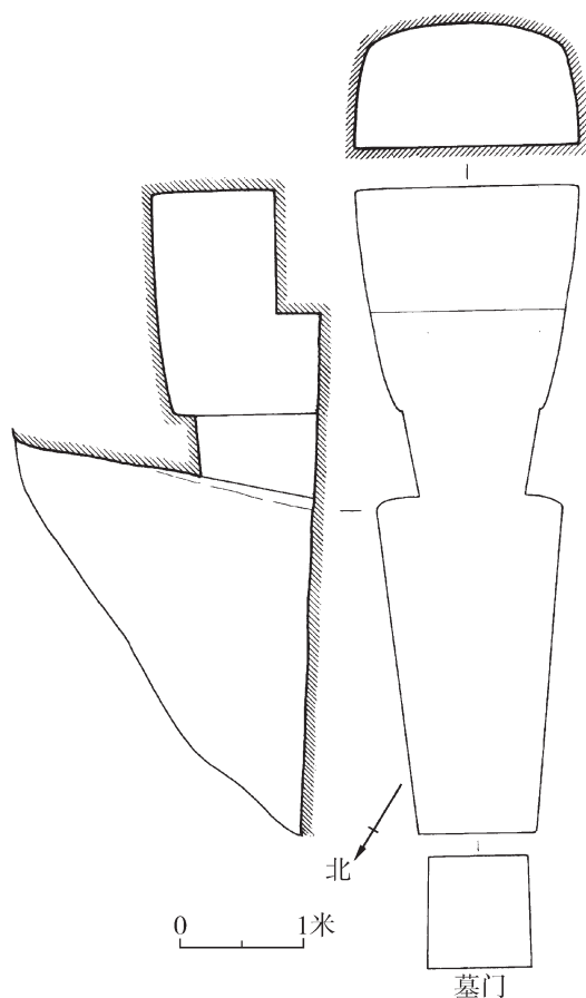
图一四 M9 平、剖面图
