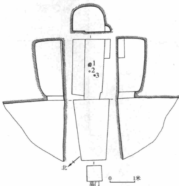
图二〇 M12平、剖面图
