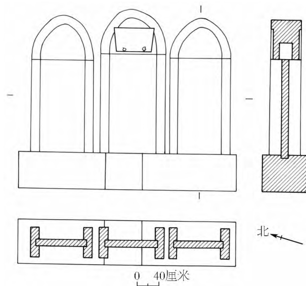
图六 1 至 3 号石刻平、立、剖面图
