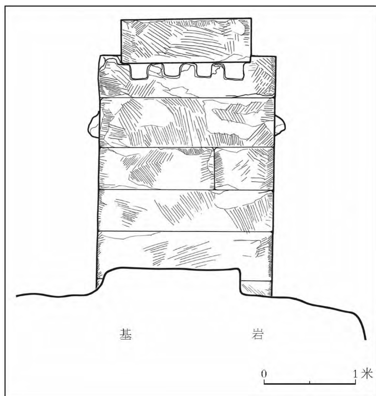
图五 1号桥址立面图
