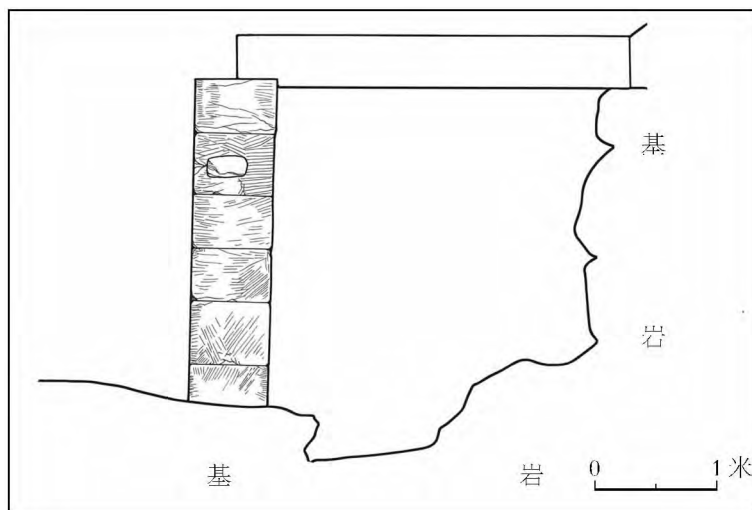
图四 1号桥址立面图
