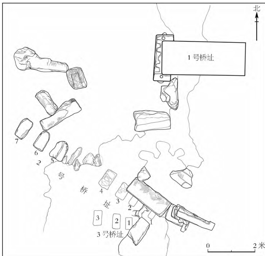
图三 1至3号桥址平面图
