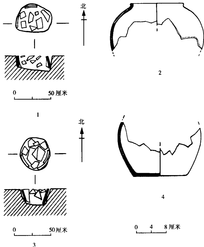
图三十五 WM6、WM4 平剖面图及瓮棺
