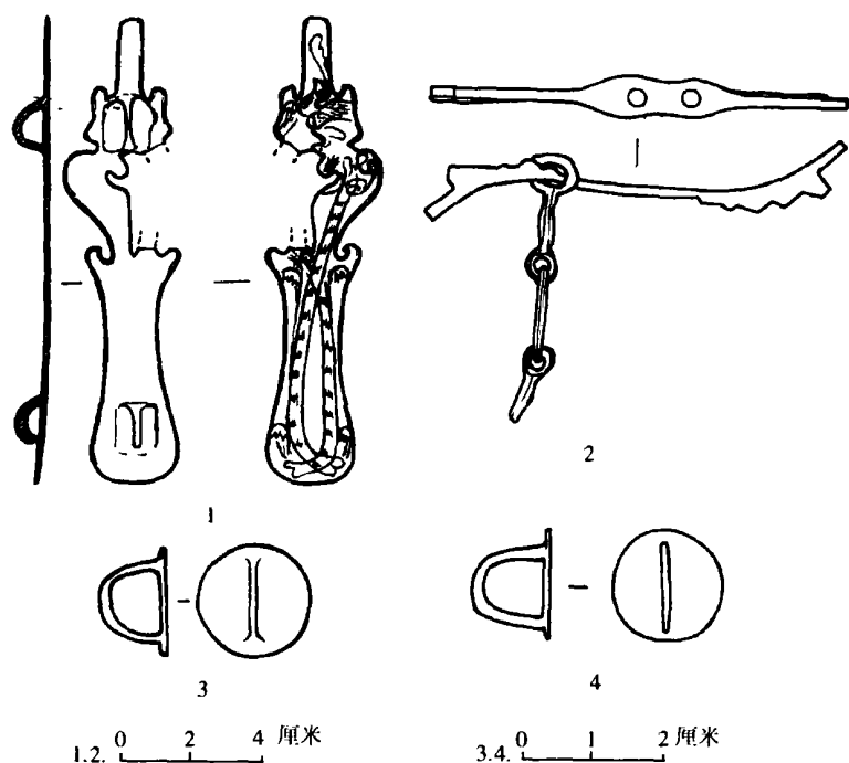
图十四 M1出土青铜器
