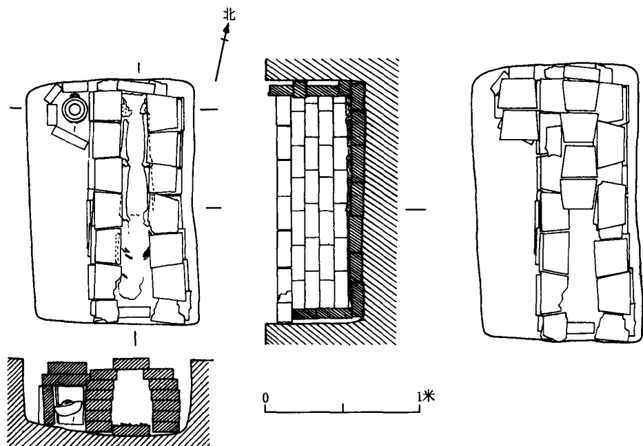
图二十九 M9 平剖面图
