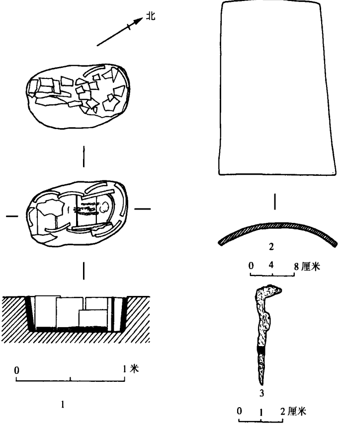
图三十四 WM3 平剖面图及出土器物 1.WM3 平剖面图 2.WM3 瓦室板瓦 3.WM3 出土铁钉
