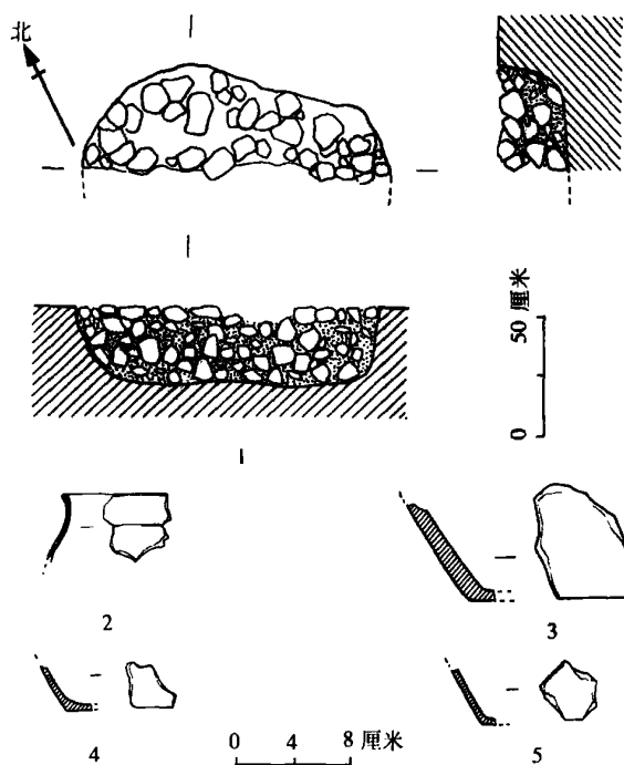
图十一 H5平剖面图及出土陶器
