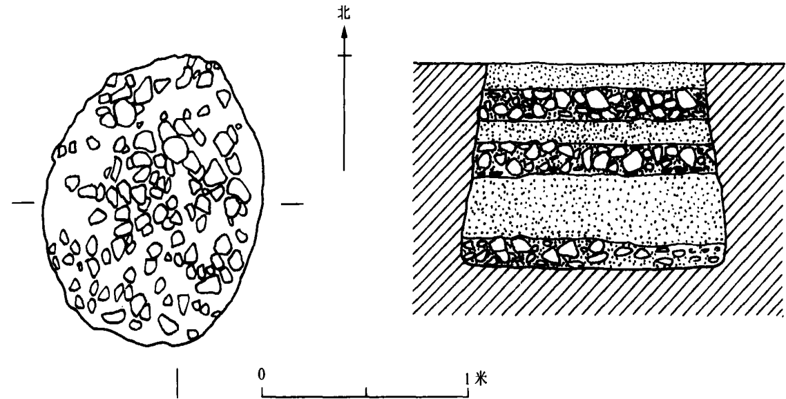
1.H2 剖面图及②层平面图
