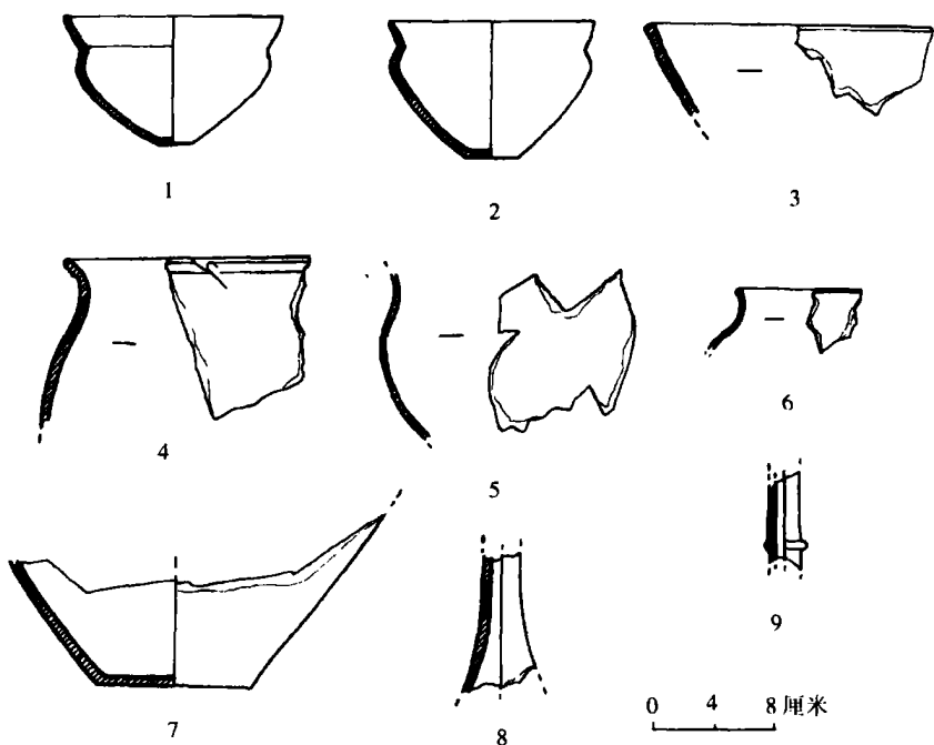
图十二 H4出土陶器组合图
