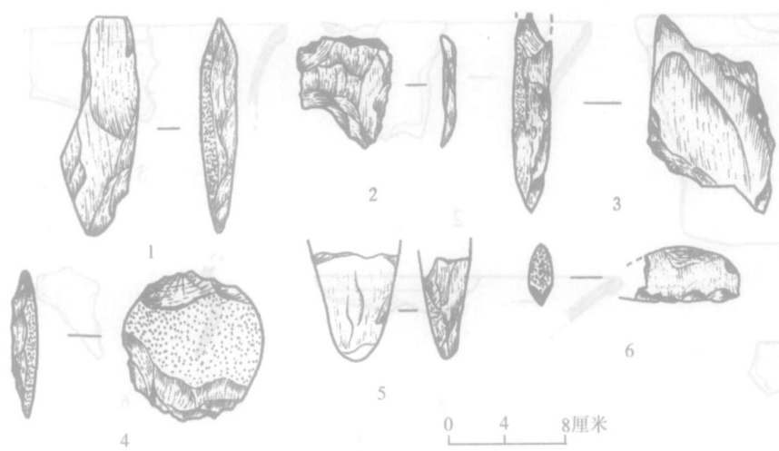
图七 H2②(第一积石层)出土石器 H2②层出土石器(H2②:14、15、16、17、18、19)
