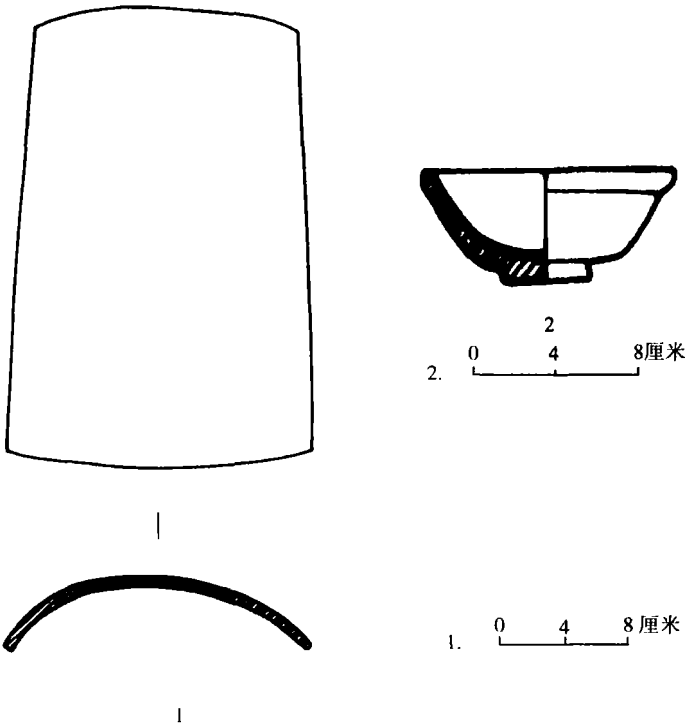
图三十一 M6 出土板瓦及釉陶碟 1. 板瓦(M6:2) 3. 釉陶碟(M6:1) (均 1/4)
