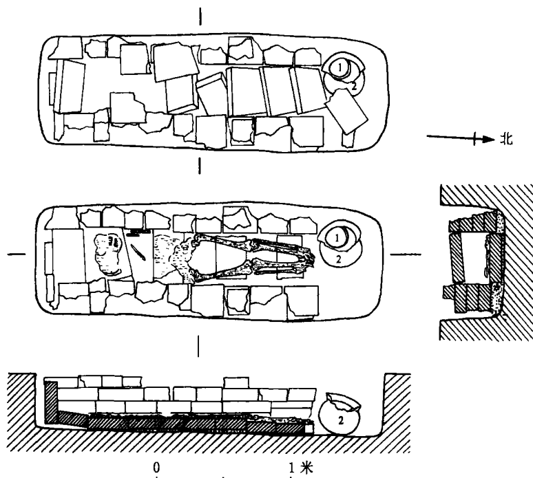
图二十六 M8 平剖面图
